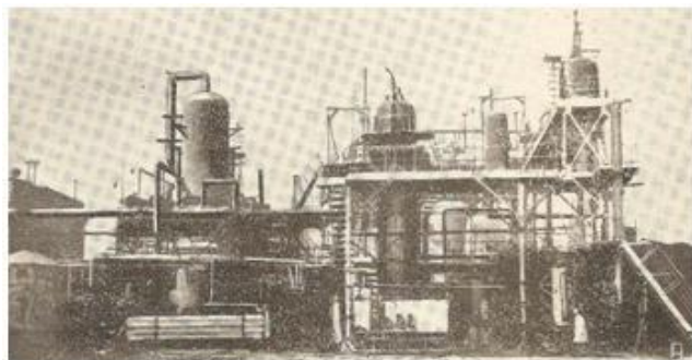
Elektrik stansiyası üçün dünyada ilk dəfə Bakıda Tikilmiş "Dəniz suyunun termokinəvi üsulla
